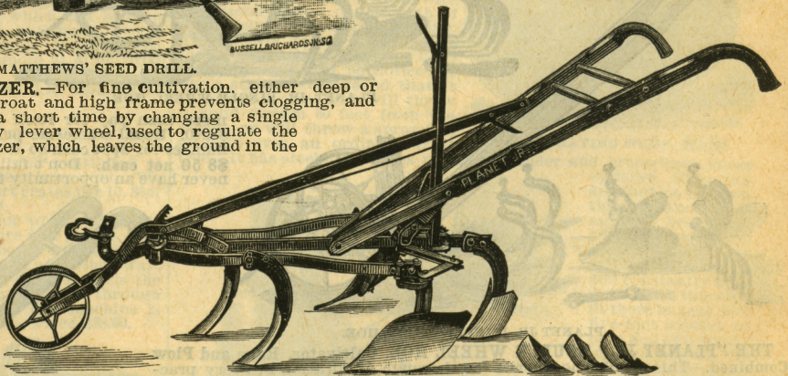
PLANET JR. NO. 6 HORSE HOE.
